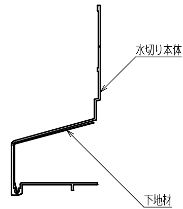
A-A断面図
