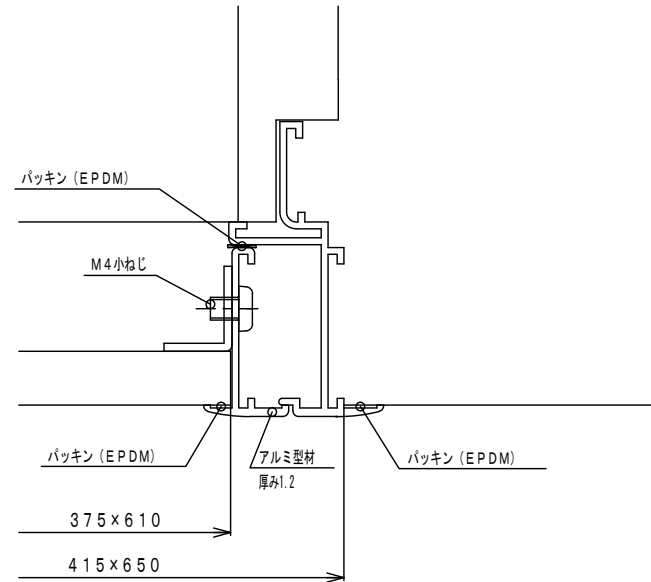
断面拡大図 S=1/1
