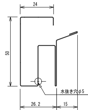
A-A断面図
