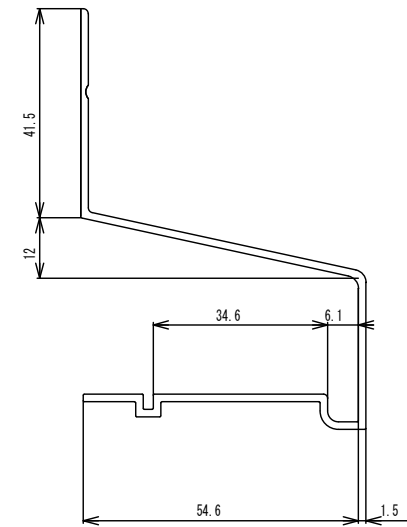
断面詳細図 S=1/1
