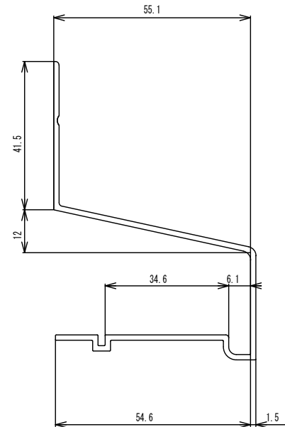
断面詳細図 S=1/1
