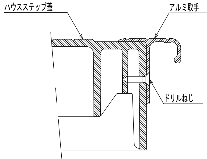
取付断面図
