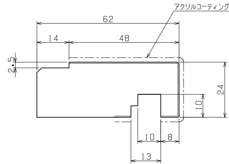
横枠 断面図 (SCALE 1/1)
