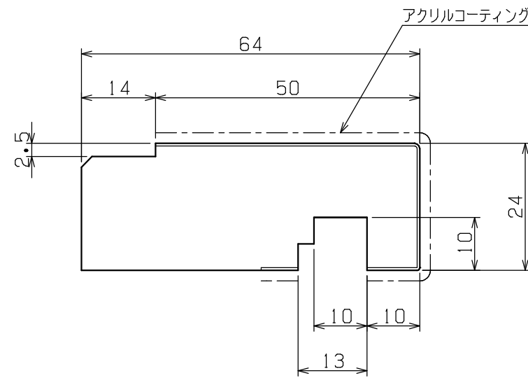
縦枠 断面図 (SCALE 1/1)
