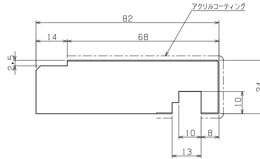
横枠 断面図 (SCALE 1/1)
