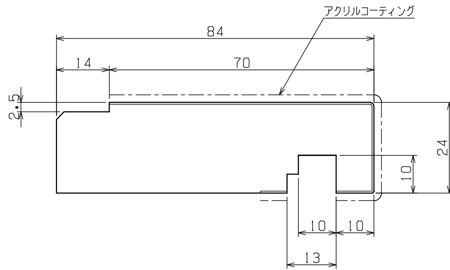
縦枠 断面図 (SCALE 1/1)
