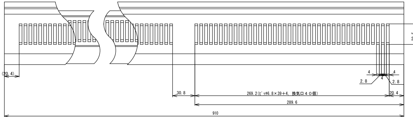
鋼板製 軒天換気材 詳細図 (S : 1 / 2)
