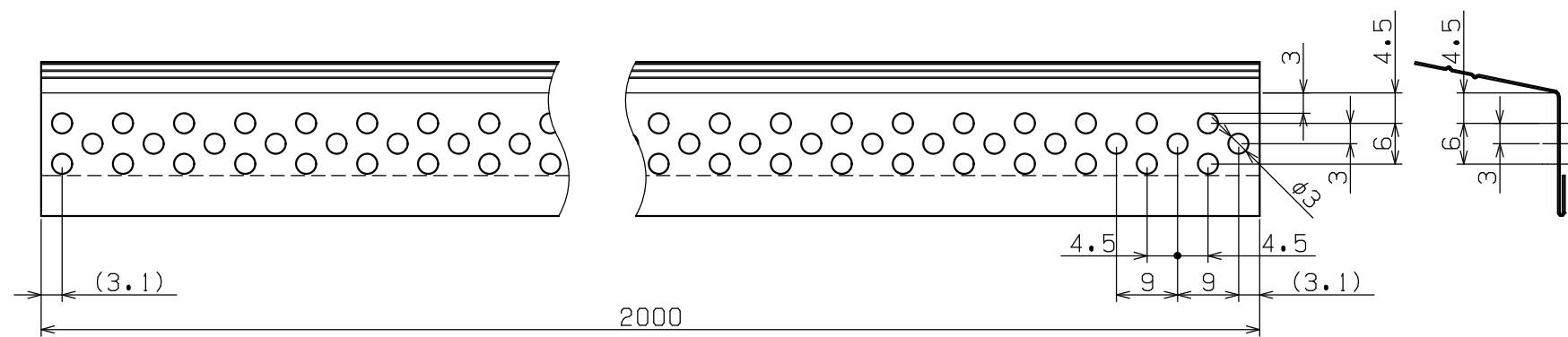
A矢視図
