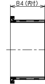
■A-A断面図
