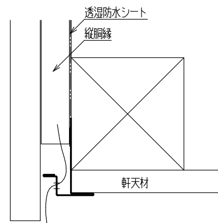
■納まり図 (S=1/2)
