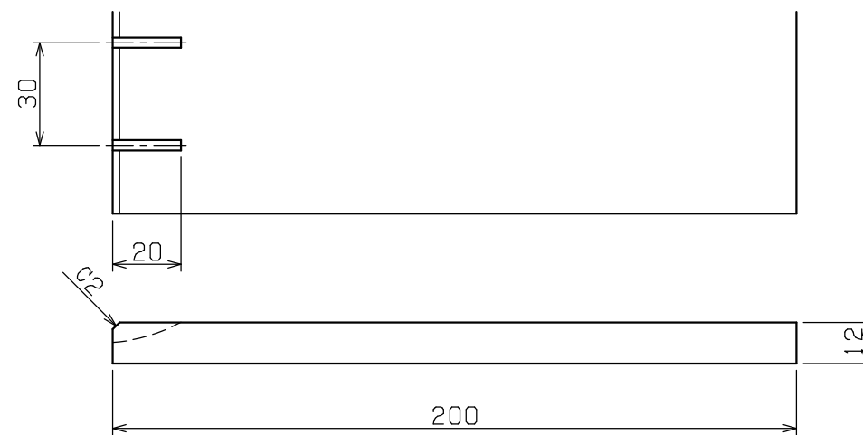
下地材 断面図 (SCALE 1/2)
