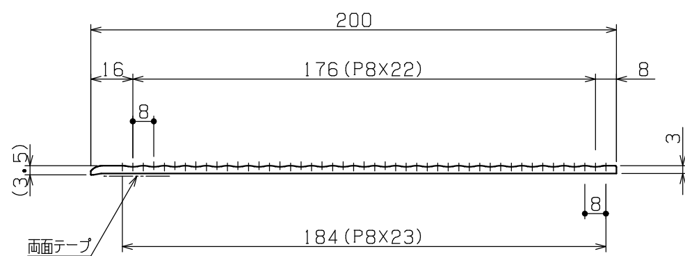
化粧下枠 断面図 (SCALE 1/2)
