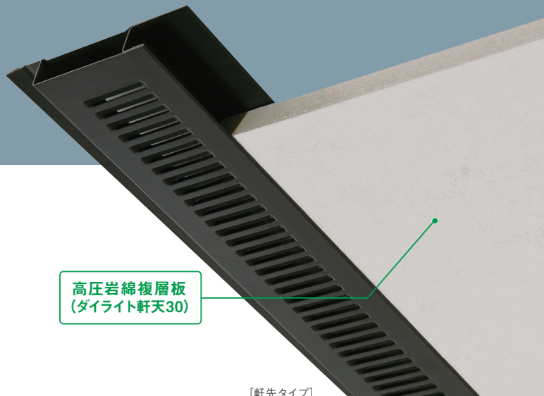
[軒先タイプ]
