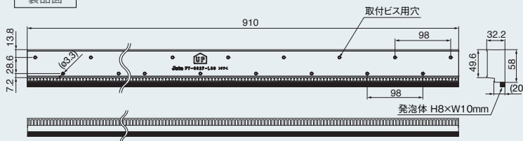
製品図
