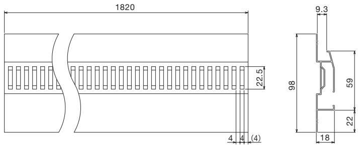
製品図
