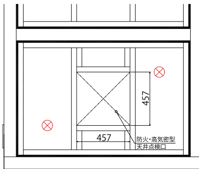
■ 床伏図 (防火・高気密型天井点検口)
