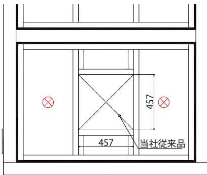
■ 床伏図 (当社従来品)
