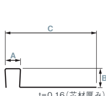
片ハット製品図
