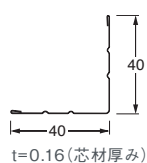
捨て入隅製品図
