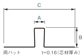
両ハット製品図
