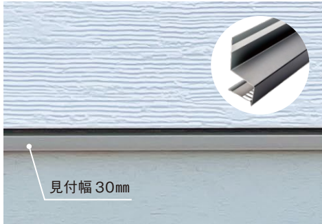
寸法図
