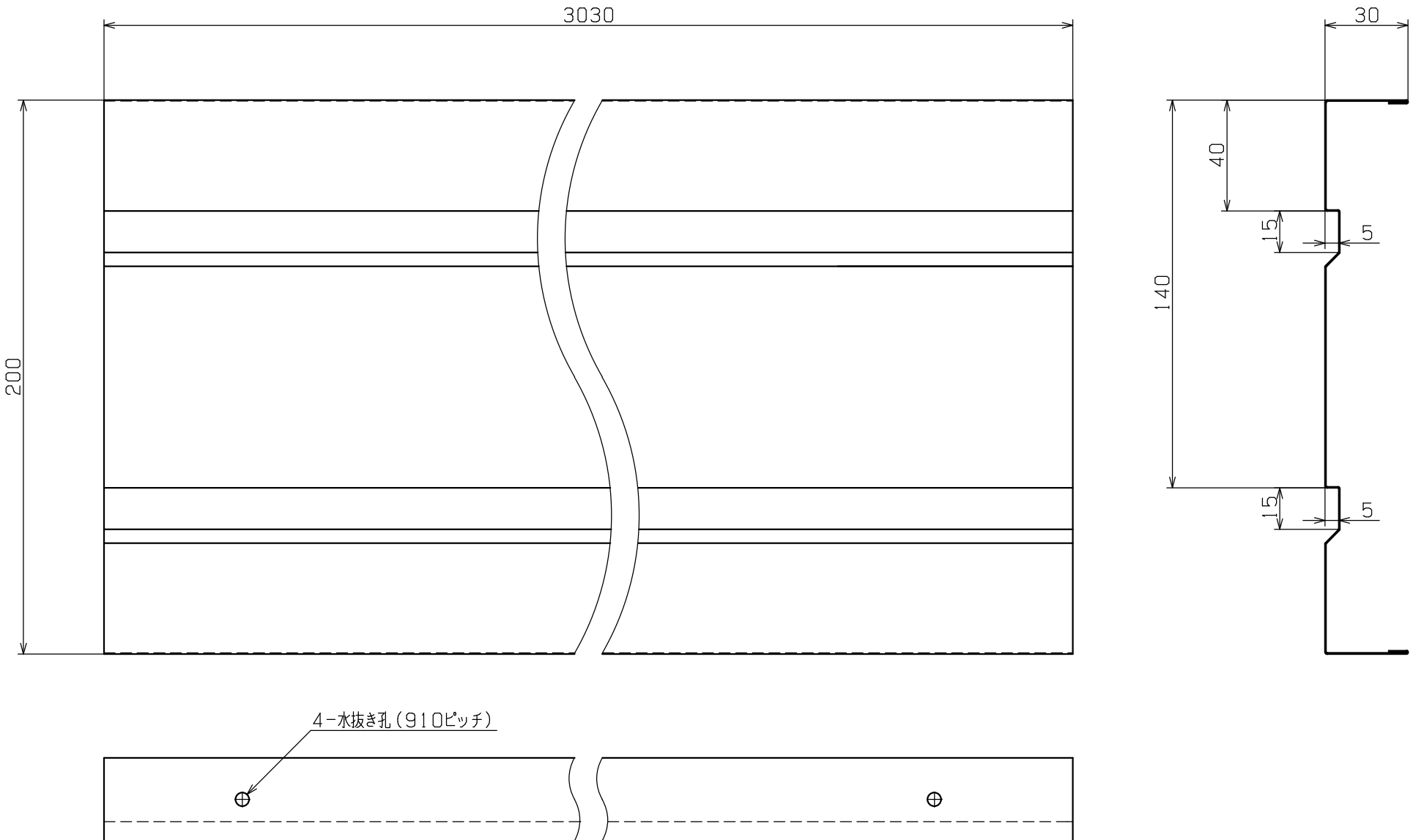
■製品図（S=1/2）
