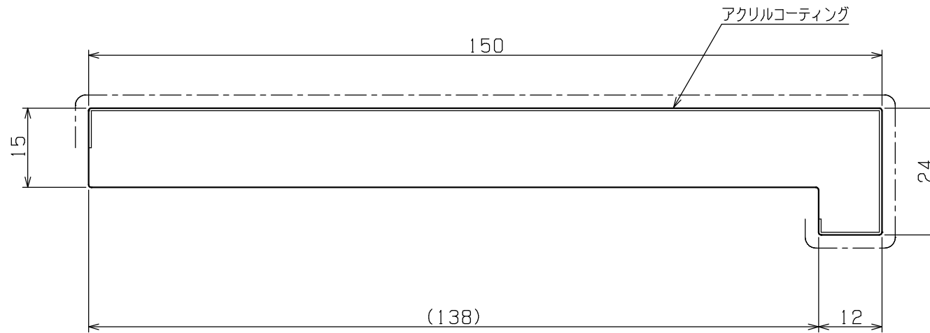
断面図 詳細 (SCALE 1/1)
