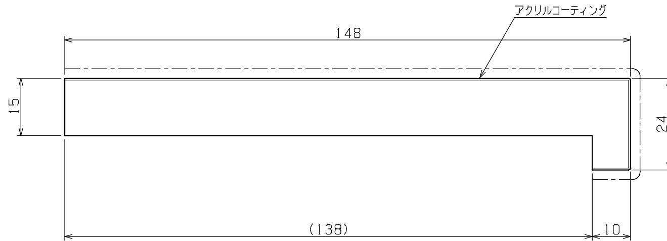
断面図 詳細 (SCALE 1/1)
