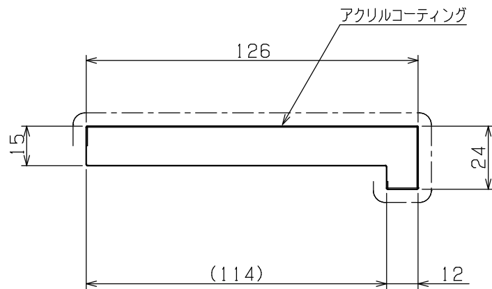
縦杵 断面図 (SCALE 1/2)
