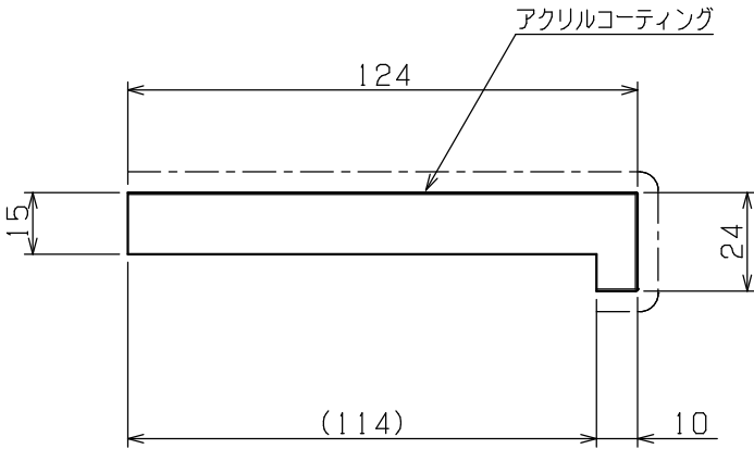
上枠 断面図 (SCALE 1/2)
