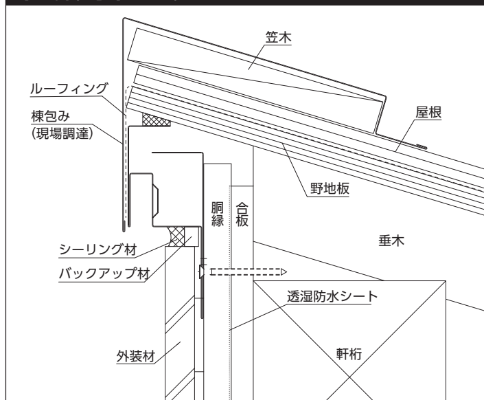
水上側 (3寸勾配まで)
