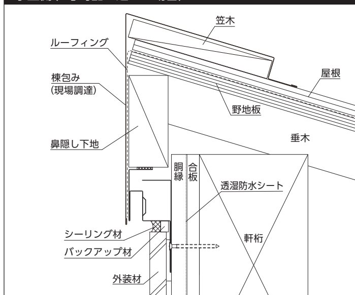
水上側 (3寸勾配を超える場合)
