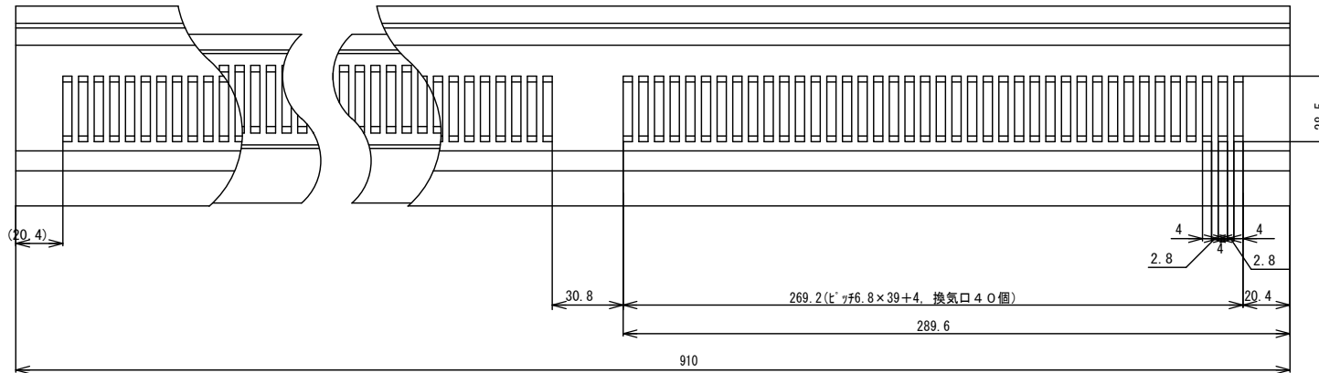
鋼板製 軒天換気材 詳細図 (S : 1 / 2)
