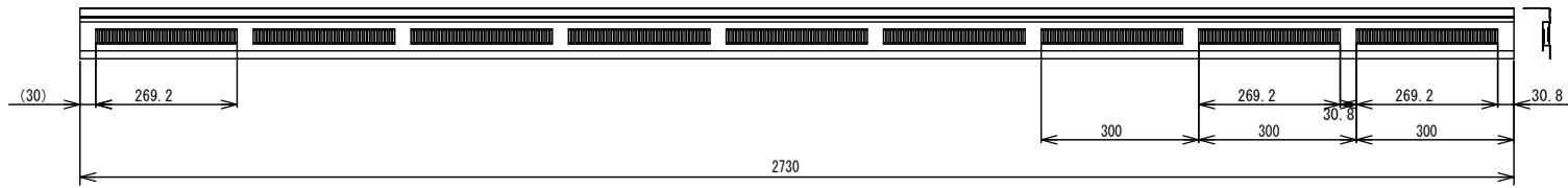
鋼板製 軒天換気材 詳細図 (S : 1/10)
