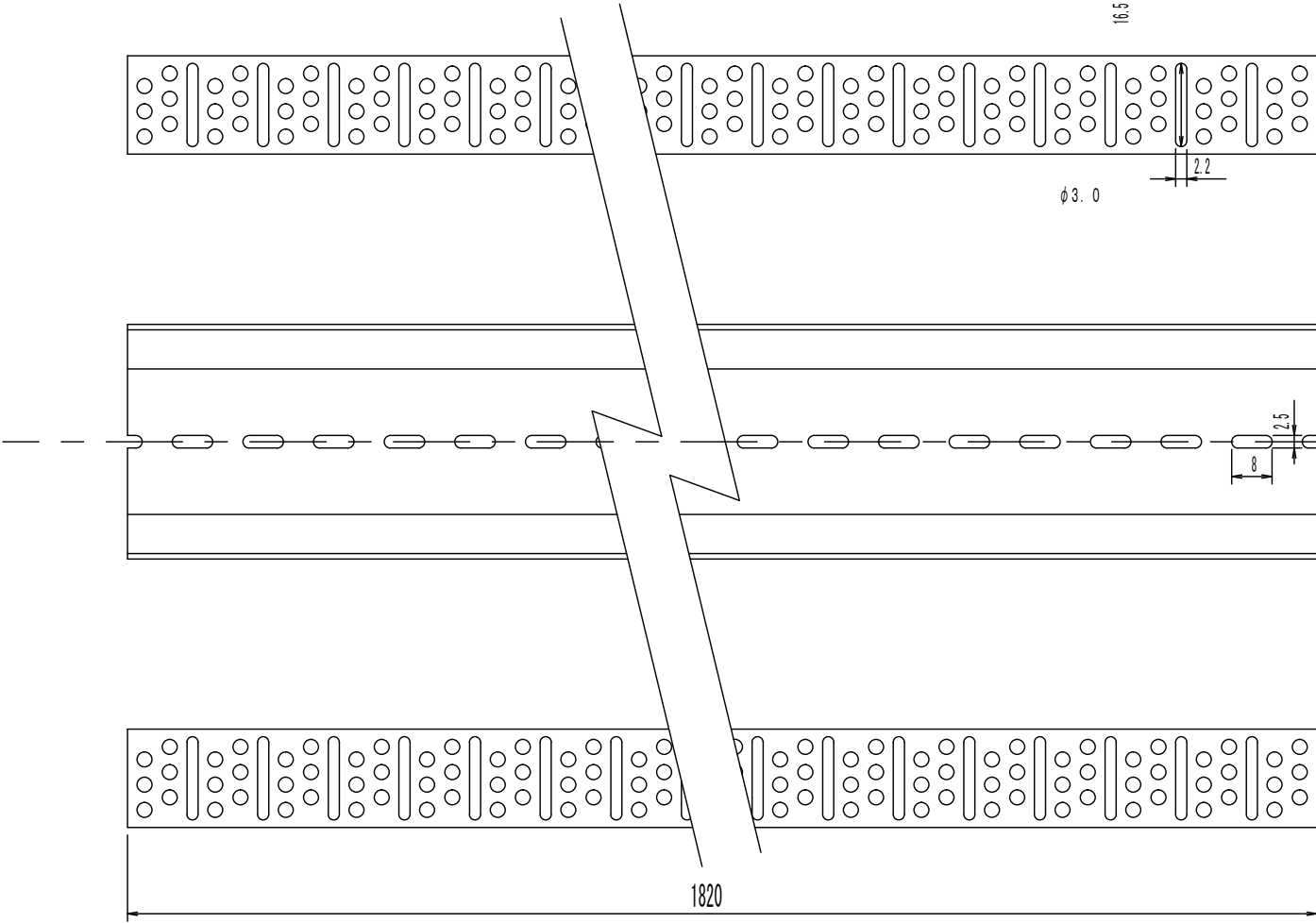
B矢视图
