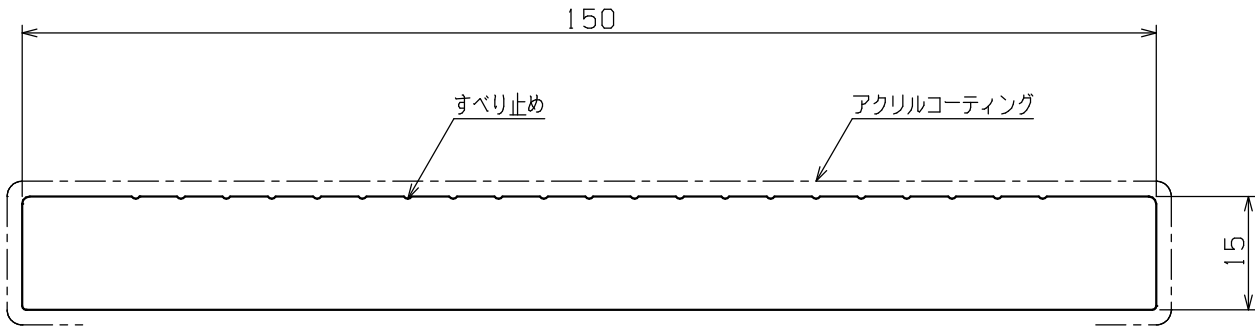
断面 詳細図 (SCALE 1/1)
