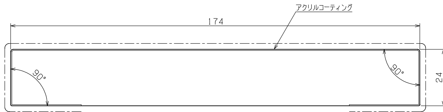
断面図 詳細 (SCALE 1/1)
