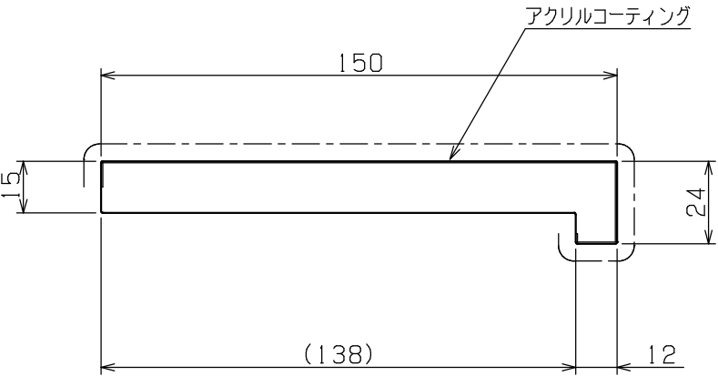
縦枠 断面図 (SCALE 1/2)
