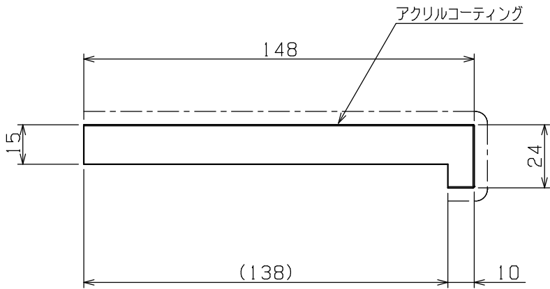
上枠 断面図 (SCALE 1/2)
