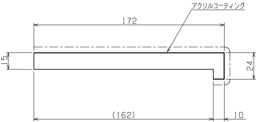
上枠 断面図 (SCALE 1/2)
