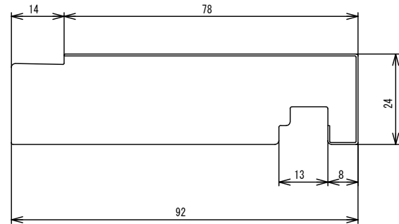
横枠 1本入
