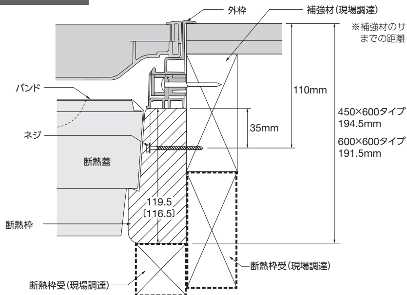
標準納まり図 〈施工例〉
