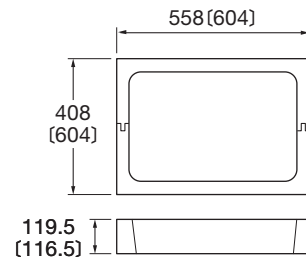
●断熱枠セット図
