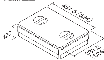
●断熱蓋図
