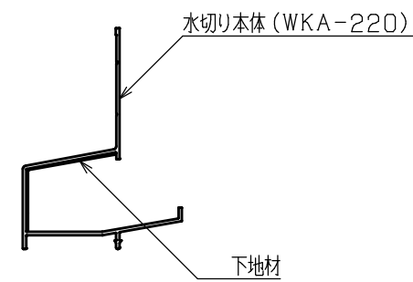
A-A断面図
