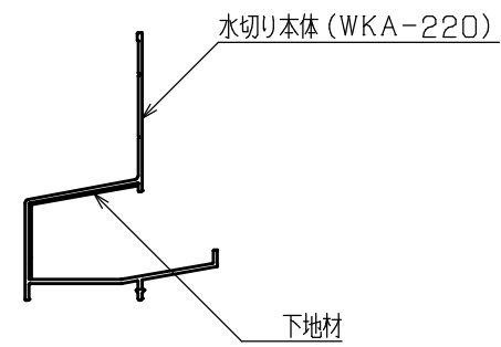
A-A断面図
