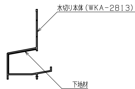
A-A断面図
