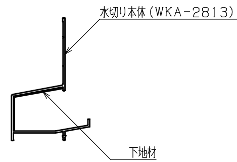
A-A断面図
