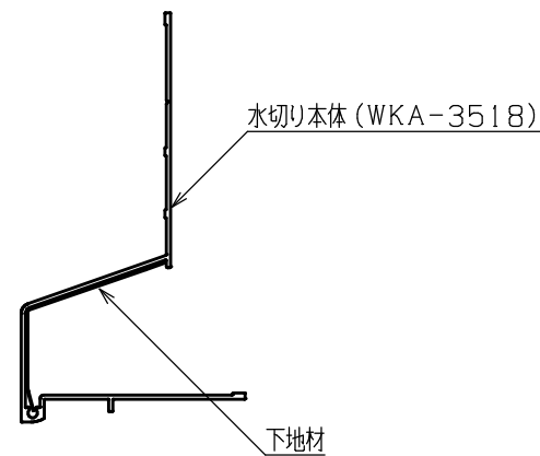
A-A断面図
