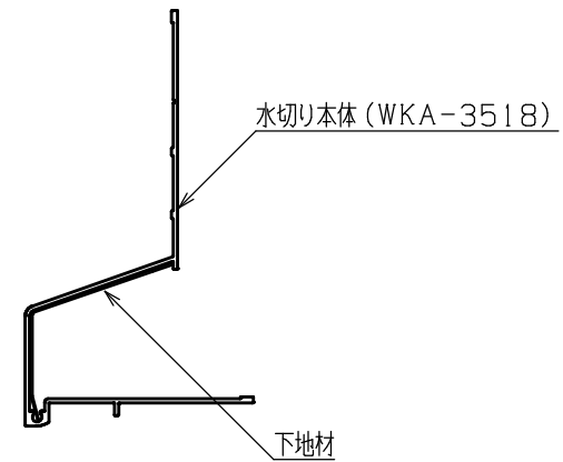
A-A断面図
