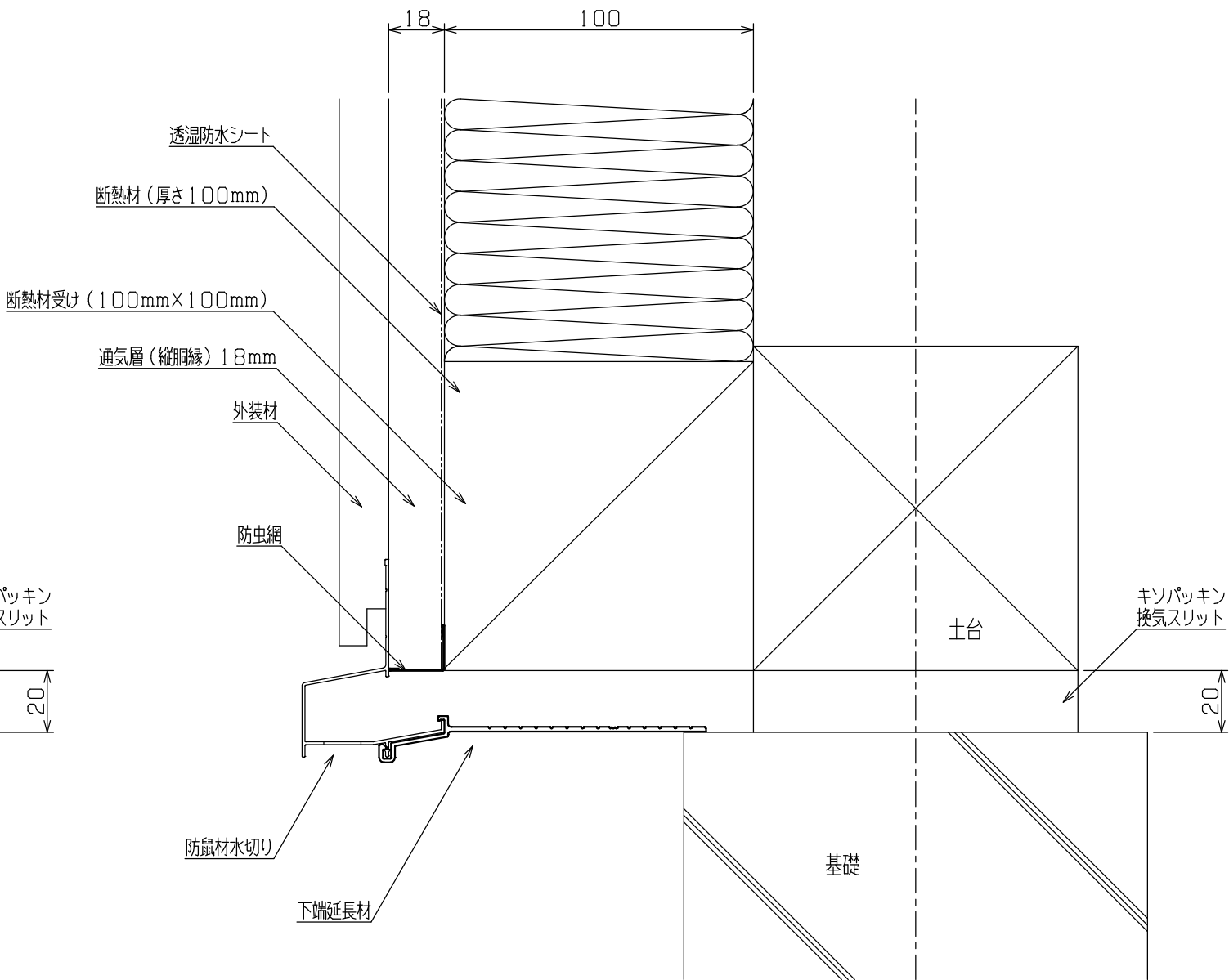
断熱材厚さ100mmの場合
