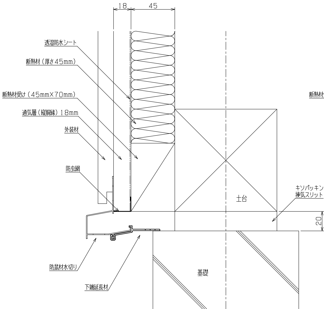
断熱材厚さ45mmの場合
