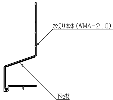
A-A断面図
