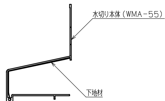
A-A断面図
