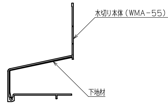
A-A断面図
