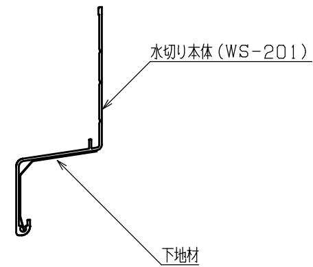
A-A断面図
