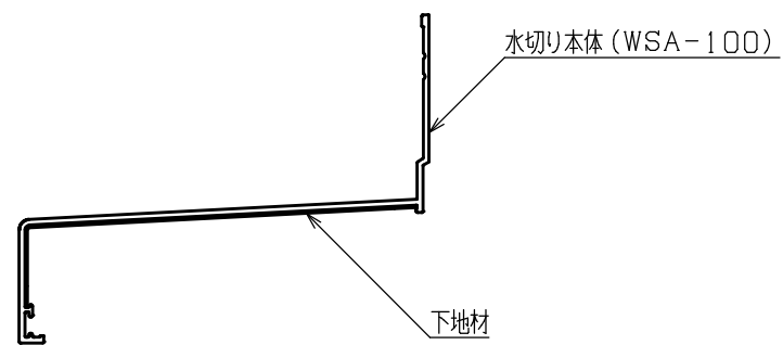
A-A断面図
