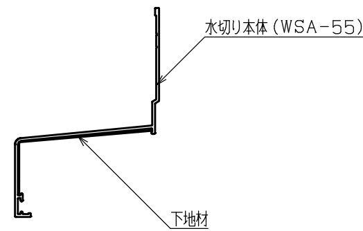
A-A断面図
