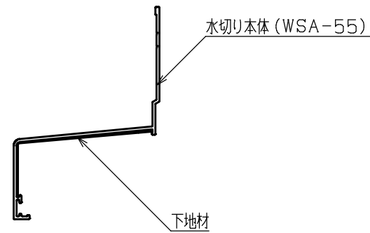
A-A断面図
