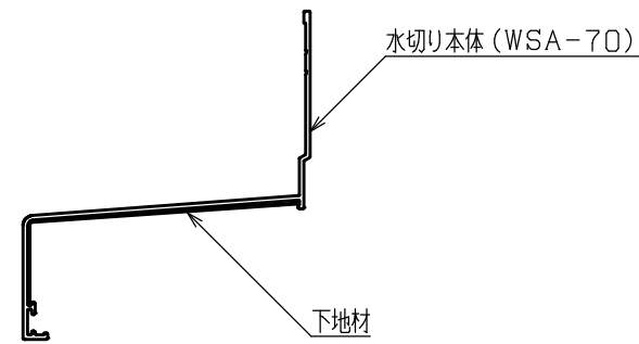
A-A断面図
