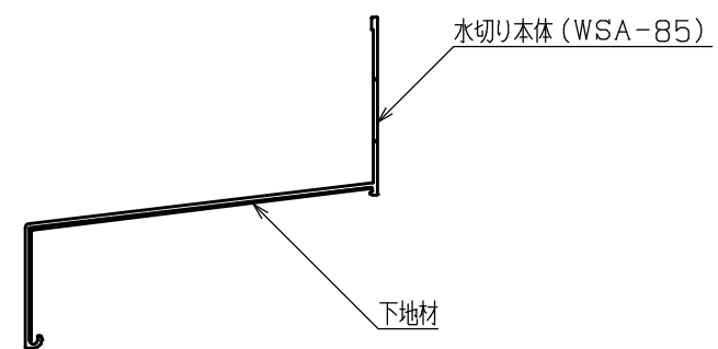
A-A断面図
